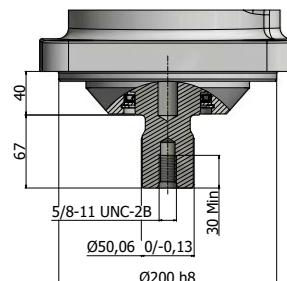
Shaft code S, -220
