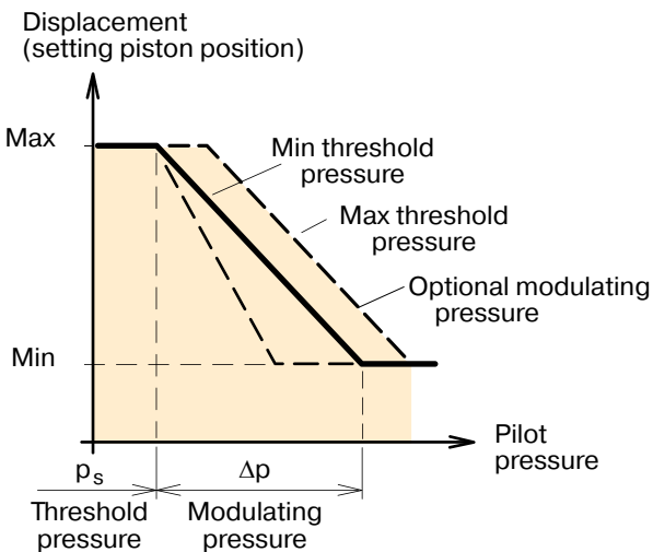
HP diagram.
