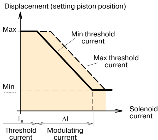
EP diagram.
