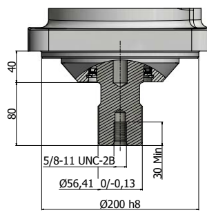
Shaft code S, -270
